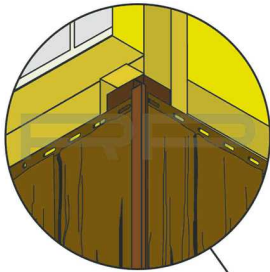
PR3527 U-Profil (2x) bei Innenecken
