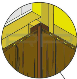
PR3527 U-Profil (2x) bei Innenecken
