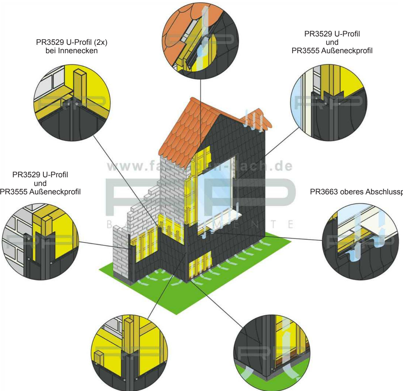
PR3555 Außeneckprofil
